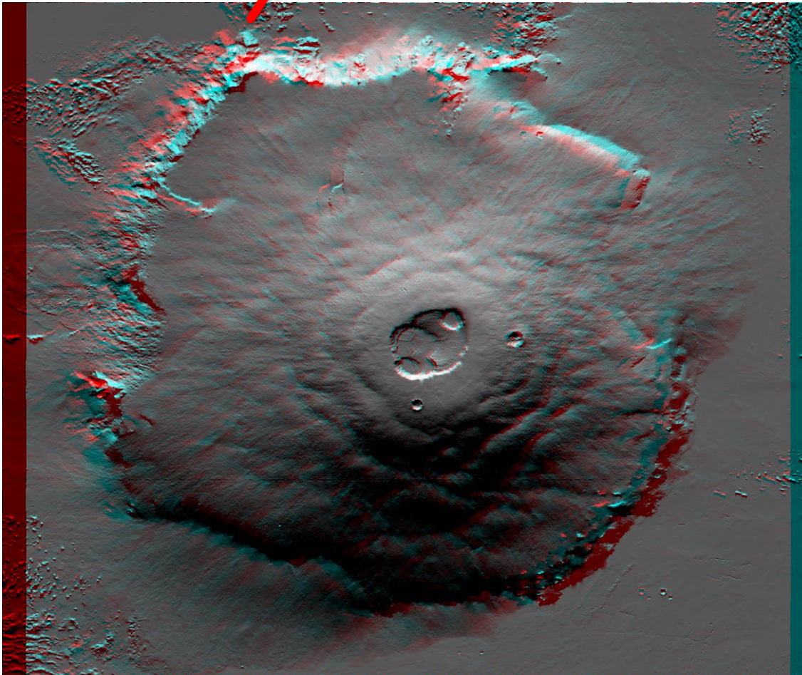
Anáglifo da região do vulcão Olympus Mons | Marte Dados: Mars Global Surveyor MOLA MEGDR 128
